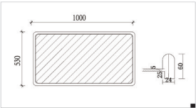
TOPM0102 矩型1000浴镜
