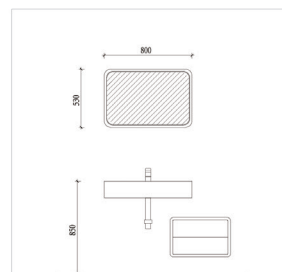
TOP 03 系列组合一 TOP0301+TOPM0101+TOPF0201 一体盆 (TOP0301单孔800矩形挂墙一体盆) 浴镜 (TOPM0101矩形800浴镜) 边柜 (TOPF0201双抽屉550边柜)
