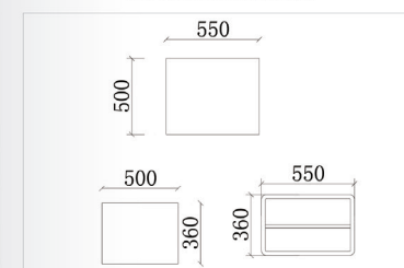
TOPF0202双层550边柜
