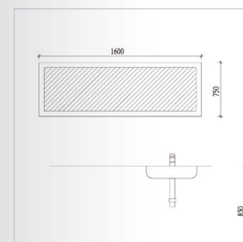
TOP 03 系列组合四 TOP0302+TOPM0301 一体盆 (TOP0302单孔1600矩形挂墙一体盆) 浴镜 (TOPM0301矩形1600浴镜)
