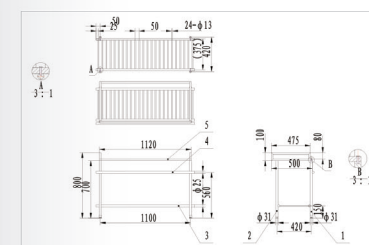
TOPF0101落地支架
