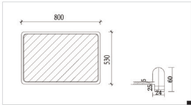
TOPM0101 矩型800浴镜
