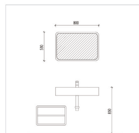
TOP 03 系列组合二 TOP0301+TOPM0101+TOPF0202 一体盆 (TOP0301单孔800矩形挂墙一体盆) 浴镜 (TOPM0101矩形800浴镜) 边柜 (TOPF0202双抽屉550边柜)
