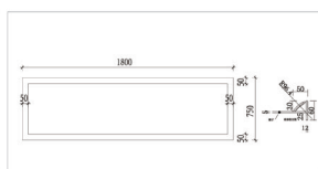
TOPM0302矩型1800浴镜
