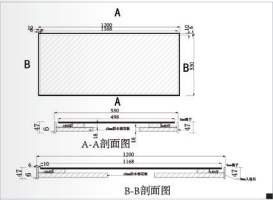
TOPM0204 矩型1200带灯浴镜
