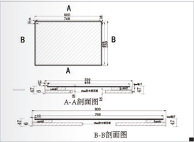
TOPM0202 矩型800带灯浴镜
